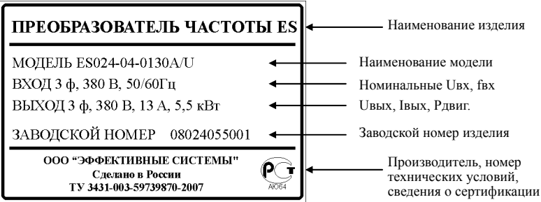
Рис. 1.2 Шильдик
