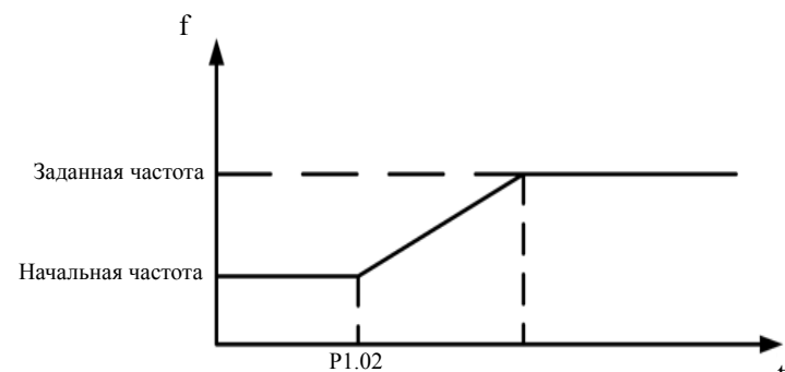
Рис. 6.3 Диаграмма запуска
