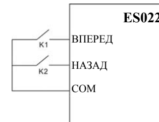
Рис. 6.10 Режим 2-проводного управления 1
