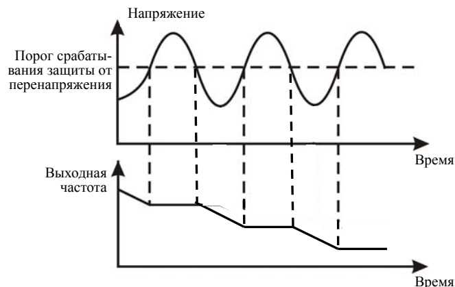
Рис. 6.28 Иллюстрация функции защиты от перенапряжения
