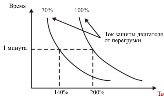
Рис. 6.27 Кривые, иллюстрирующие защиту двигателя от перегрузки
