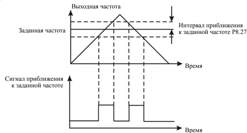
Рис. 6.19 Диаграмма сигнала приближения к заданной частоте
