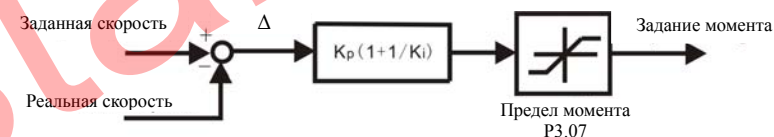
Рис. 6.6 Структура APC
