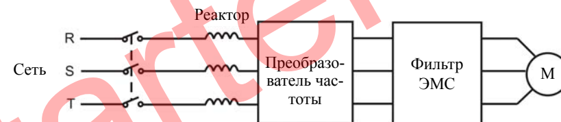
Рис. 4.13 Подключение выходных цепей
