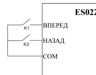
Рис. 6.11 Режим 2-проводного управления 2
