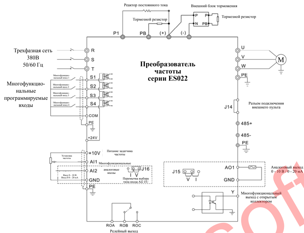
Рис. 4.11 Схема подключения
