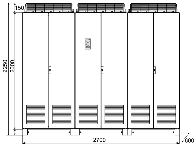
Устройство Emotron VFX48: модель 2K25 (типоразмер корпуса N) Устройство Emotron VFX69: модель 1K8 (типоразмер корпуса N69)
