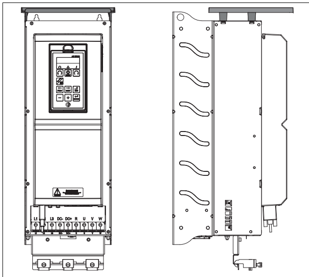
Рис. 138 Дополнительная верхняя крышка, установленная на корпусе типоразмера D2
