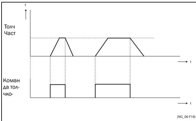
Рис. 89 Команда толчкового режима
