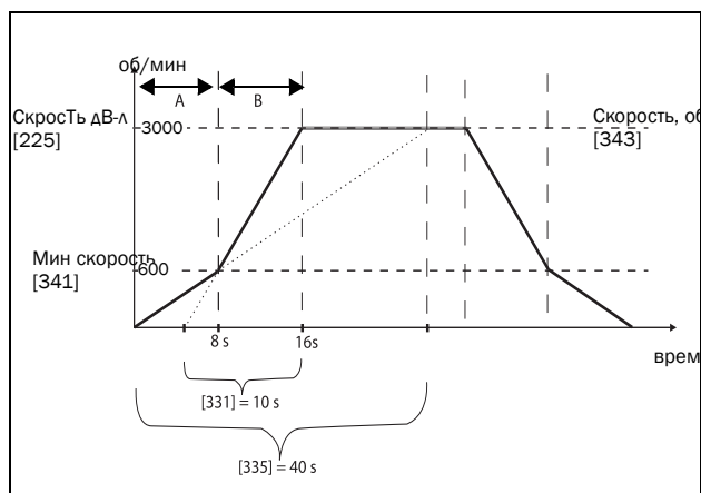
Рис. 82 Пример расчета времени разгона (графические данные не пропорциональны).
