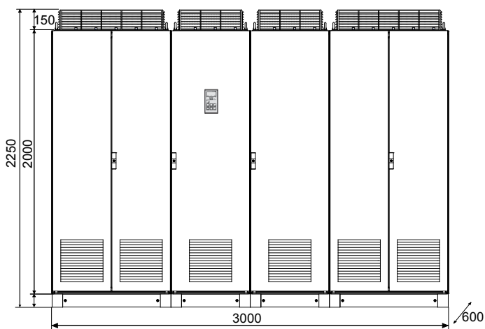
Устройство Emotron VFX48: модель 2K5 (типоразмер корпуса O) Устройство Emotron VFX69: модель 2K0 (типоразмер корпуса O69)
