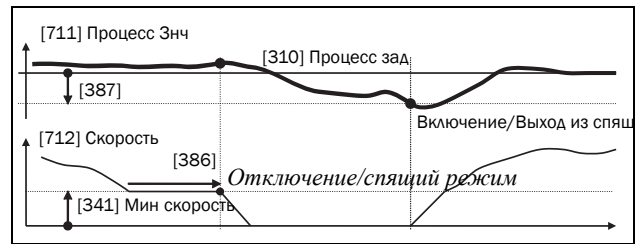
Рис. 94 Отключение/спящий режим ПИД при обычном ПИД-управлении
