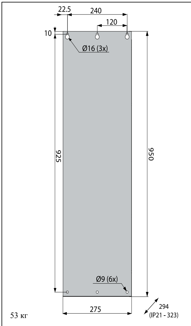
Рис. 18 Устройство Emotron VFX/ моделей 48-106 – 48-171 (типоразмер корпуса E2).
