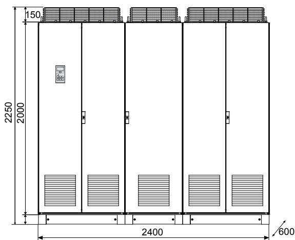
Устройство Emotron VFX48: модель 2K0 (типоразмер корпуса M) Устройство Emotron VFX69: модель 1K6 (типоразмер корпуса M69)
