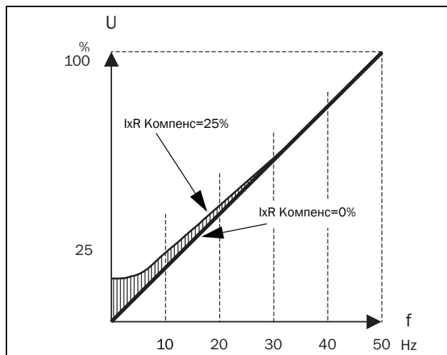
Рис. 90 IxR компенсация при линейной зависимости В/Гц
