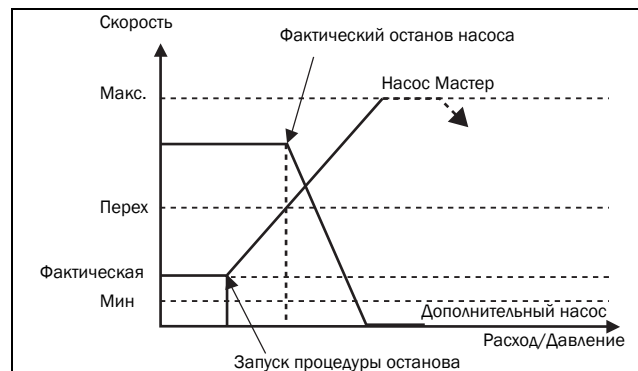
Рис. 103 Скорость перехода при останове
