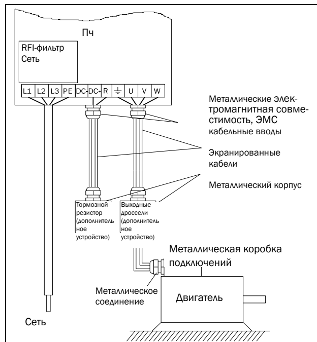
Рис. 52 Подключение кабелей двигателя и сетевого питания
