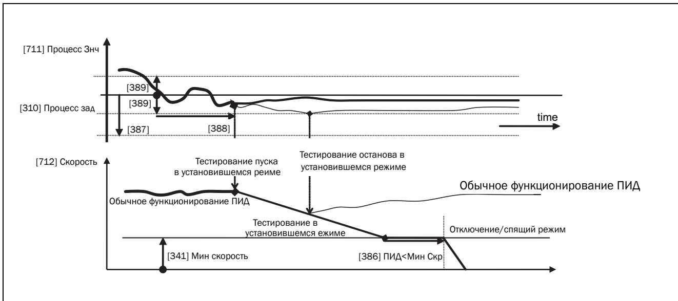
Рис. 96 Тестирование в установившемся режиме
