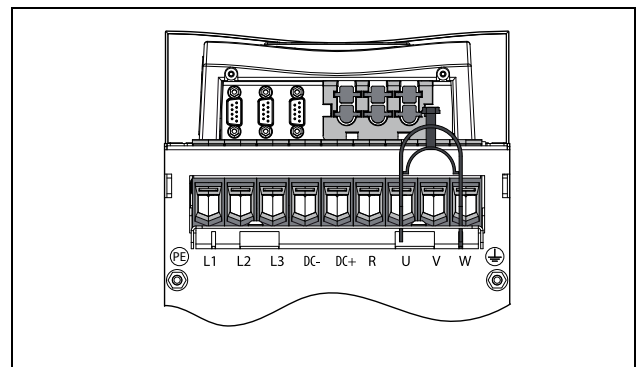
Рис. 15 Вид снизу, устройство Emotron VFX моделей от 48-060 до 48-088 (типоразмер D2), с кабельным интерфейсом для подключения электрической сети, электродвигателя, опции DC+/DC-, тормозного резистора и управления.
