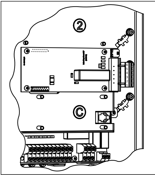
Рис. 135 Подключение опциональной платы Безопасного Останова для размера В и D.
