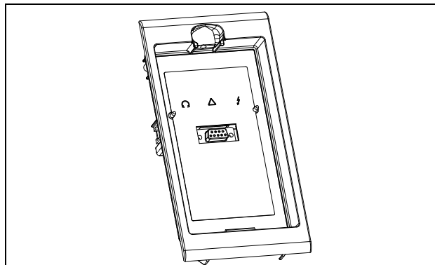
Рис. 73 Разъем RS232 под панелью управления
