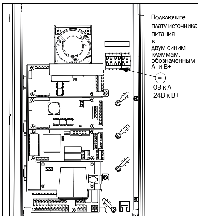
Рис. 134 Подключение опции резервного источника питания для типоразмеров D и D2
