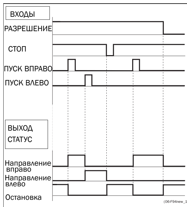
Рис. 60 Состояние входов и выходов при управлении фронтом
