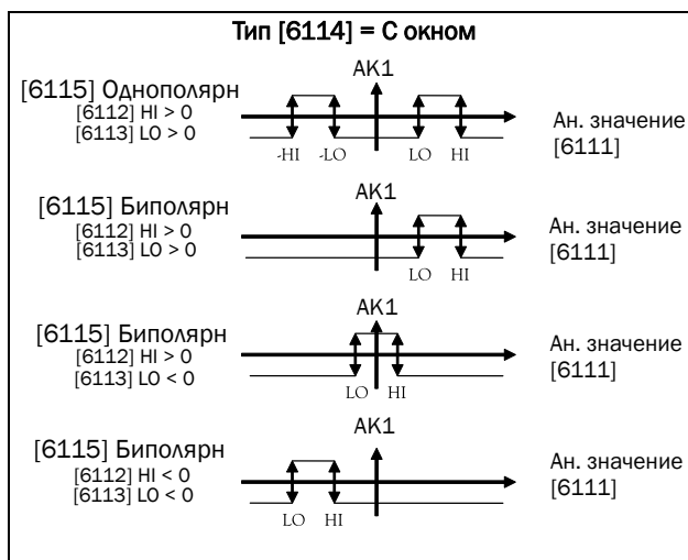
Рис. 118 Основные функции компаратора для "Тип [6114] = С окном" и "Полярн [6115]".
