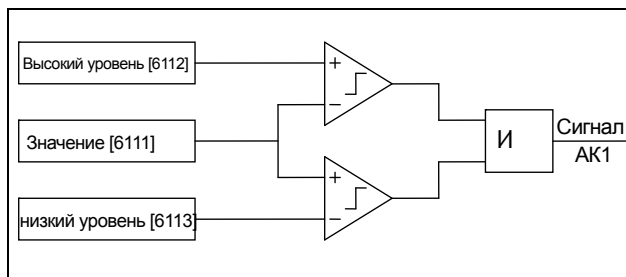
Рис. 114 Аналоговый компаратор двухпорогового типа
