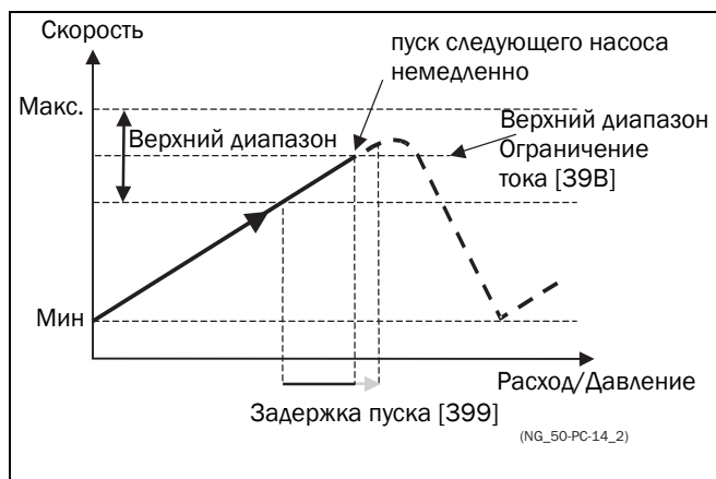
Рис. 99 Ограничение верхнего диапазона
