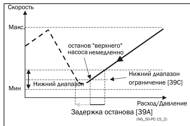
Рис. 100 Ограничение нижнего диапазона
