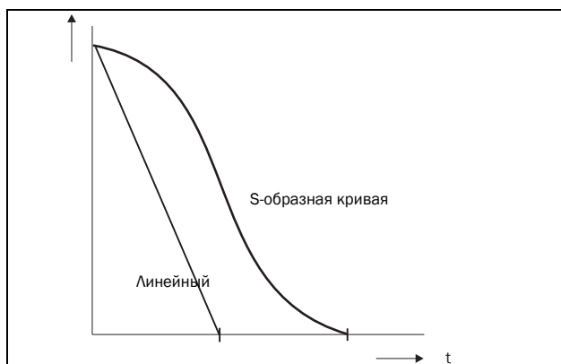
Рис. 84 Форма кривой торможения
