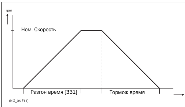
Рис. 81 Время разгона и торможения
