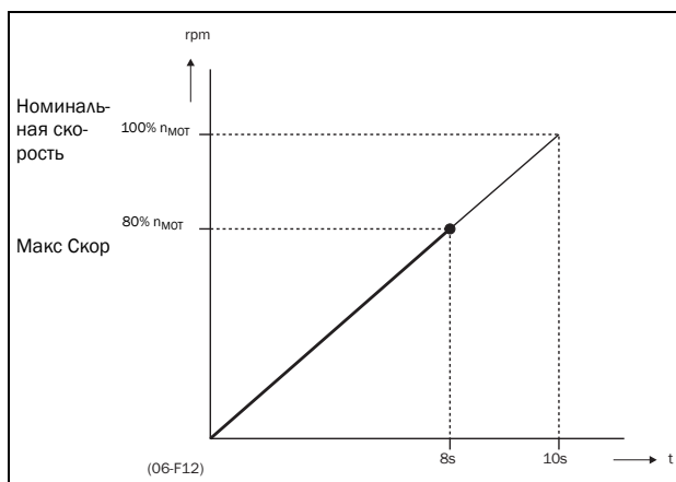
Рис. 80 Время разгона и максимальная скорость
