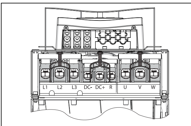
Рис. 19 Вид снизу, устройство Emotron VFX/ моделей 48-106 – 48-244 (типоразмеры корпуса E2 и F2), с кабельным интерфейсом для подключения электрической сети, электродвигателя, опции DC+/DC-, тормозного резистора и управления. (принципиальная схема)
