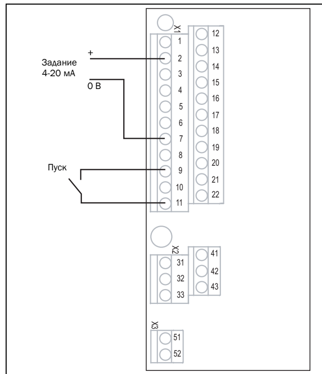
Рис. 54 Подключение
