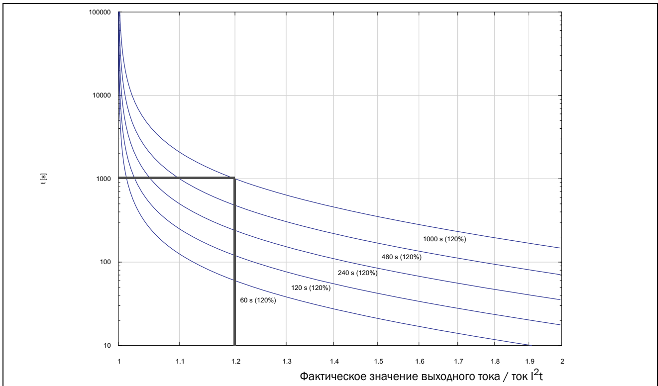
Рис. 77 Функция I^2t
