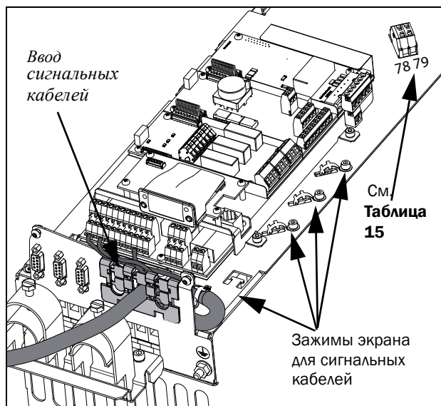
Рис. 46 Подключение кабелей управления, VFX/ модели от 48-025 до 48-045, типоразмер С2.
