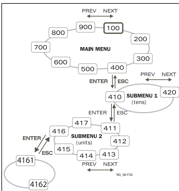
Рис. 71 Структура меню
