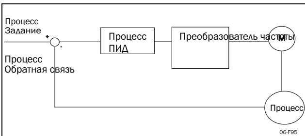
Рис. 93 Замкнутый контур ПИД-регулирования
