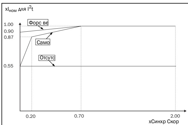
Рис. 76 Кривые I 2 t
