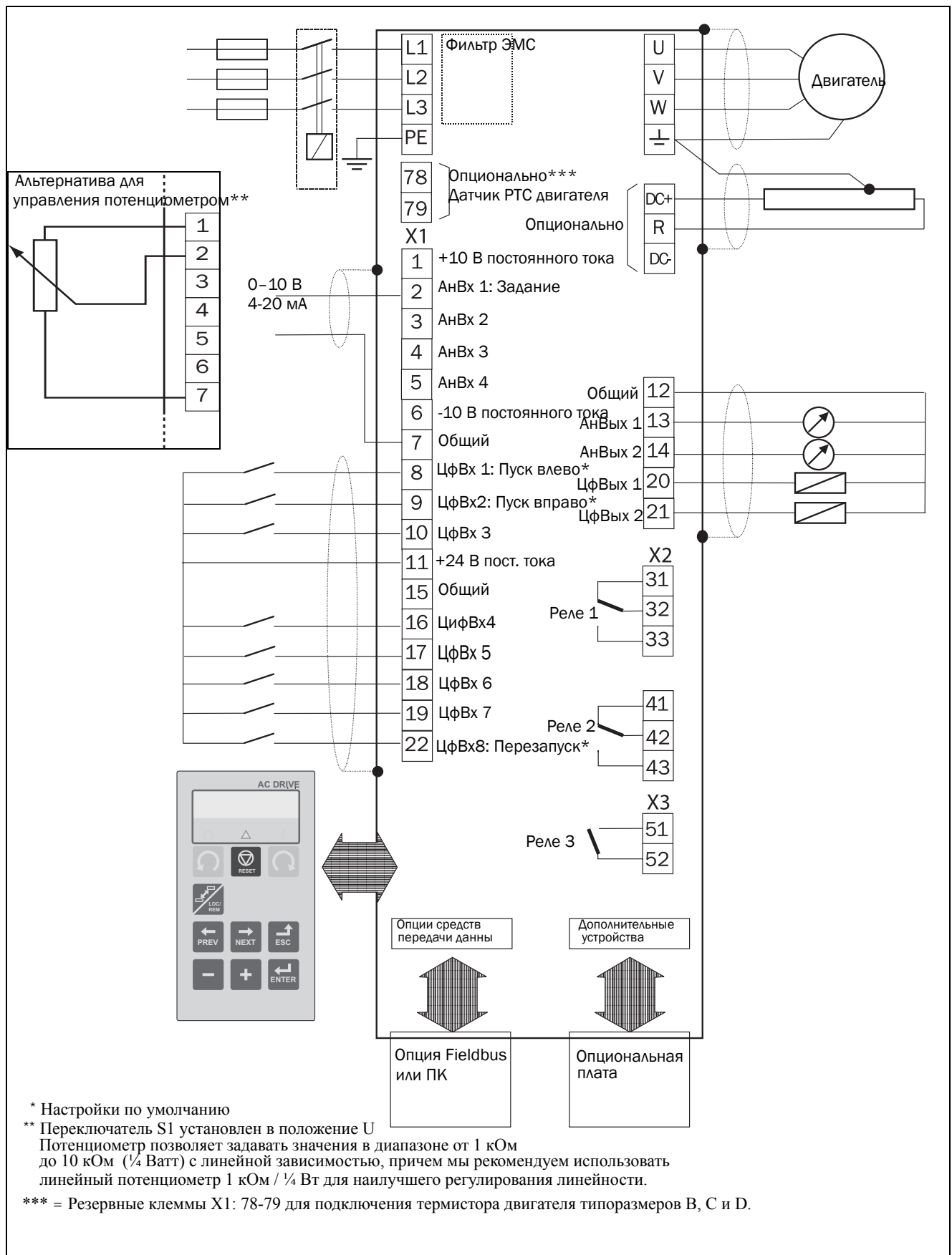
Рис. 43 Пример подключения
