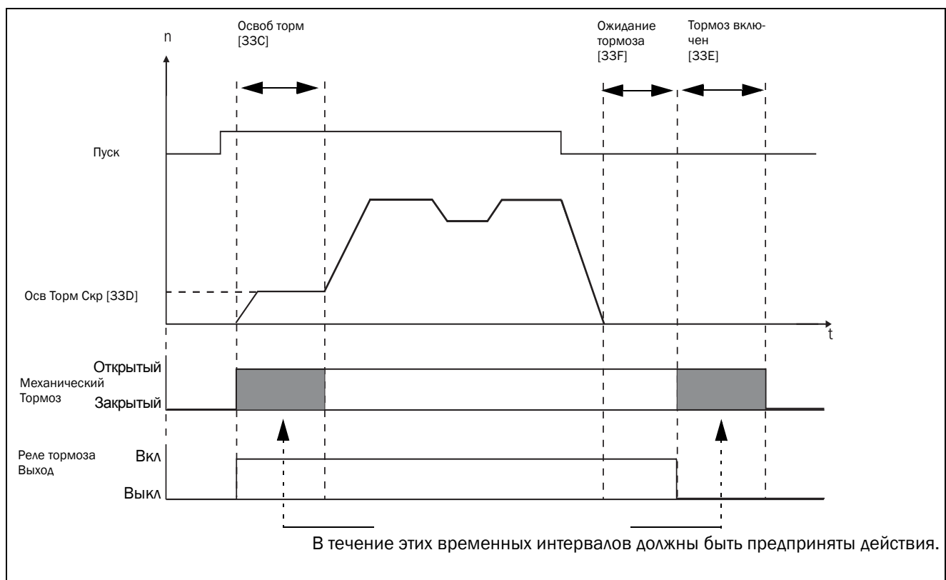
Рис. 85 Функции торможения
