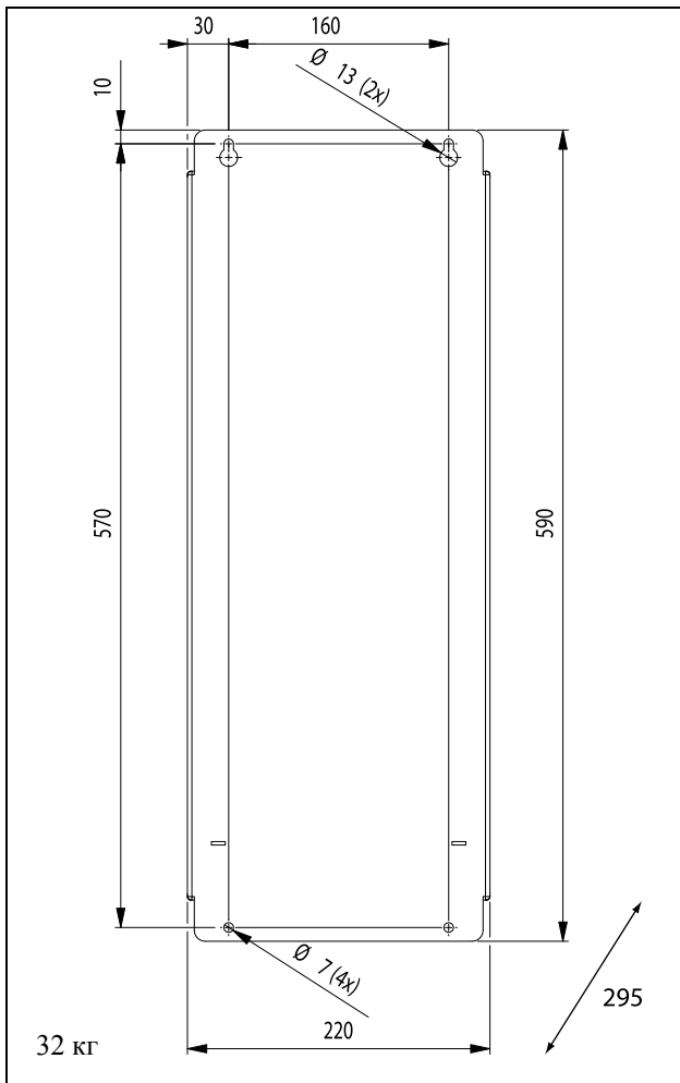
Рис. 12 Устройство Emotron VFX моделей 48/52-061 и 074 (типоразмер корпуса D)
