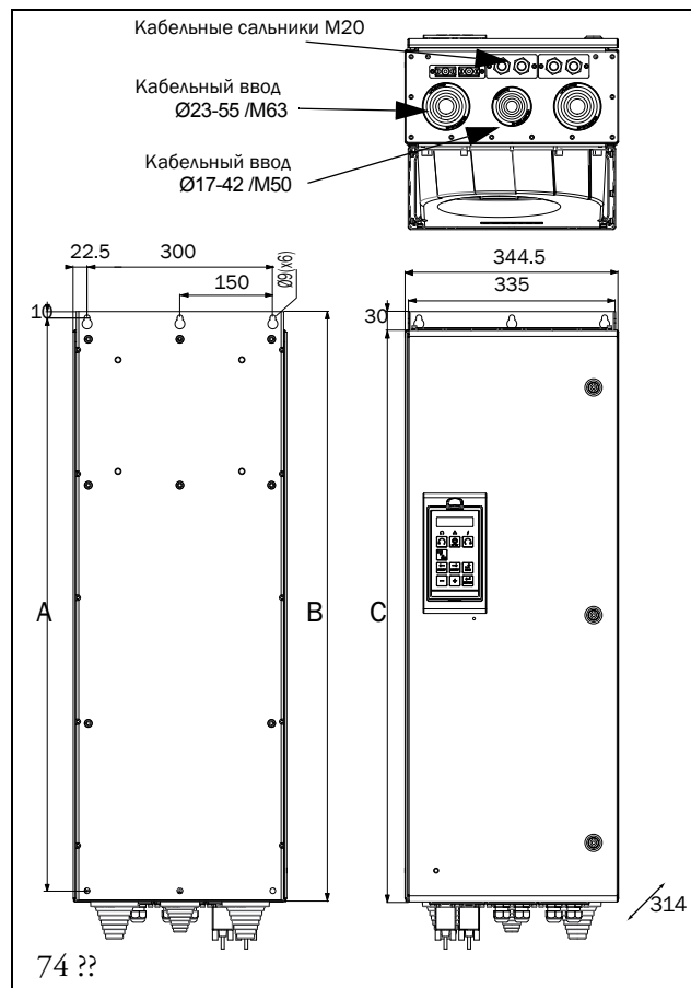
Рис. 17 Устройство Emotron VFX моделей 48-210 - 250 (типоразмер корпуса F) Устройство Emotron VFX моделей 69-90 – 200 (типоразмер корпуса F69) с кабельным интерфейсом для подключения электрической сети, электродвигателя, опции DC+/DC-, тормозного резистора и связи
