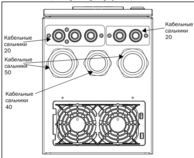
Рис. 12 Устройство Emotron VFX моделей 48/52-061 и 074 (типоразмер корпуса D)
