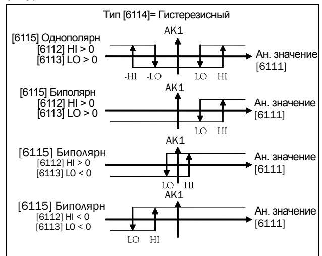
Рис. 117 Основные функции компаратора для "Тип [6114] = Гистерезис" и "Полярный [6115]".
