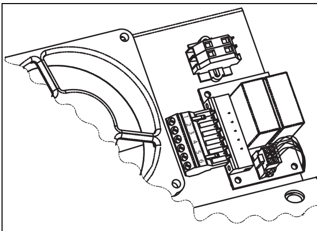
Рис. 136 Подключение опциональной платы Безопасного Останова для размера E и больше.
