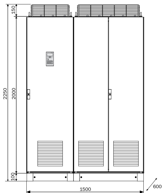
Устройство Emotron VFX48: модели 1K15 – 1K25 (типоразмер корпуса KA) Устройство Emotron VFX69: модели 905 – 995 (типоразмер корпуса KA69)
