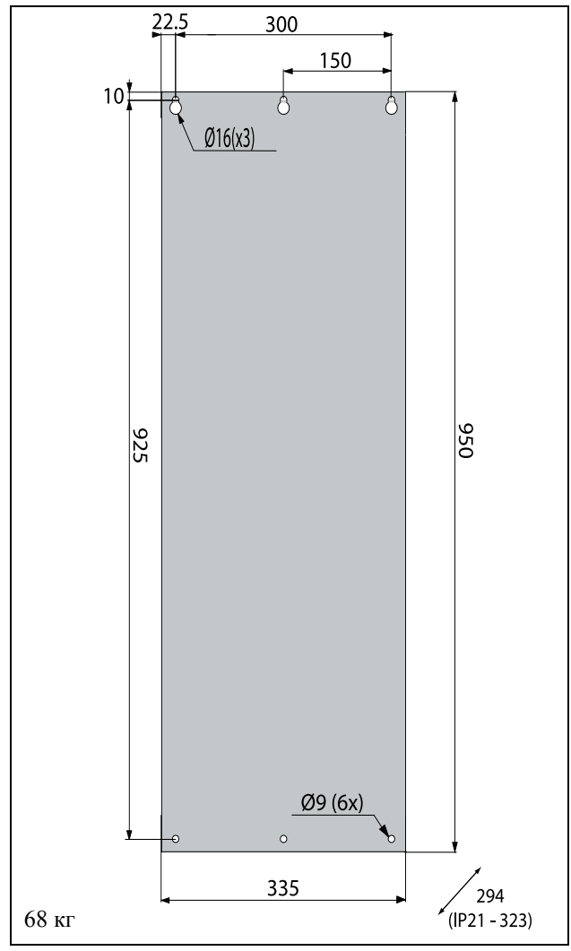
Рис. 20 Устройство Emotron VFX/ моделей 48-205 – 48-244 (типоразмер корпуса F2).
