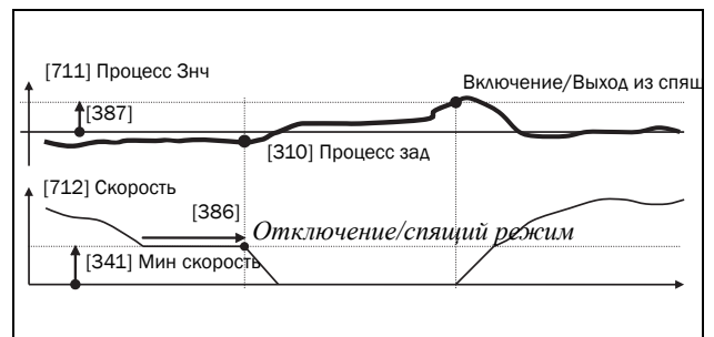
Рис. 95 Отключение/спящий режим ПИД при обратном ПИД-управлении
