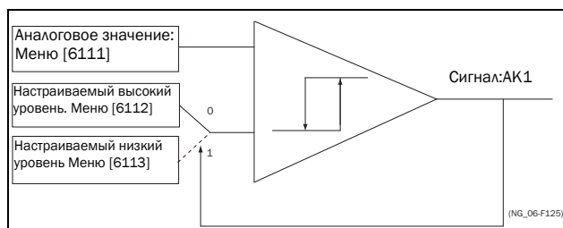
Рис. 113 Аналоговый компаратор гистерезисного типа
