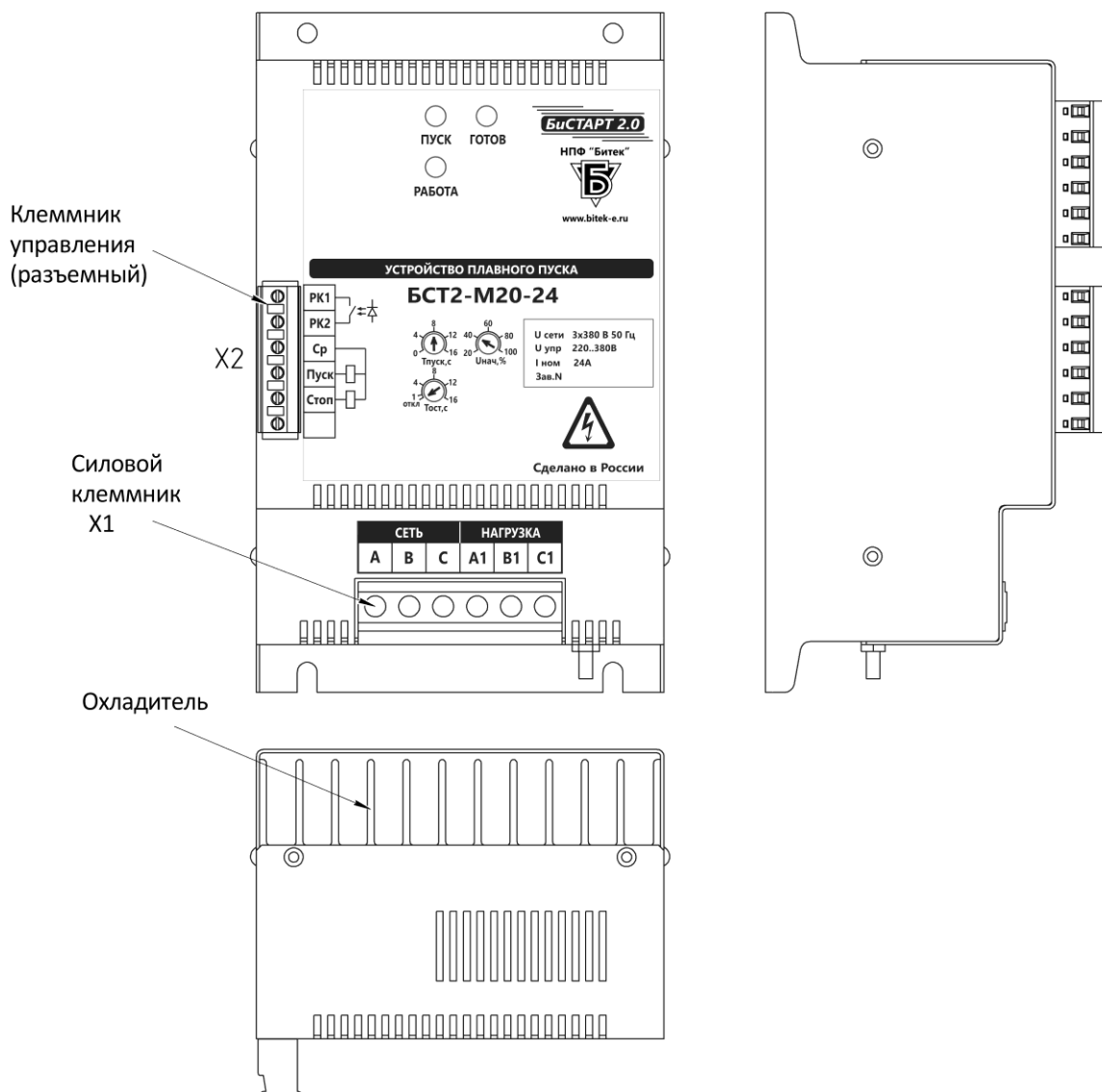
Рисунок 1 - Внешний вид пускателя БСТ2-M20-24
