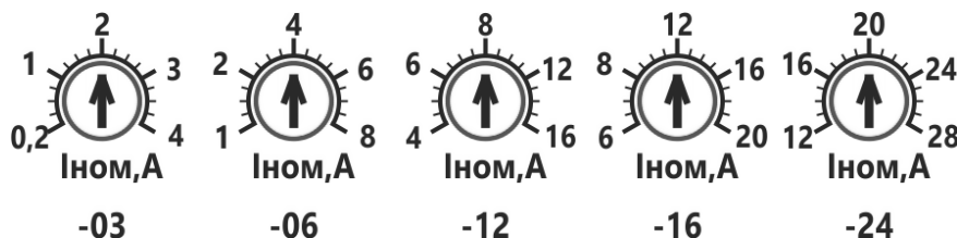
Рисунок 6 Диапазоны настройки Ином для моделей 03А, 06А, 12А, 16А, 24А
