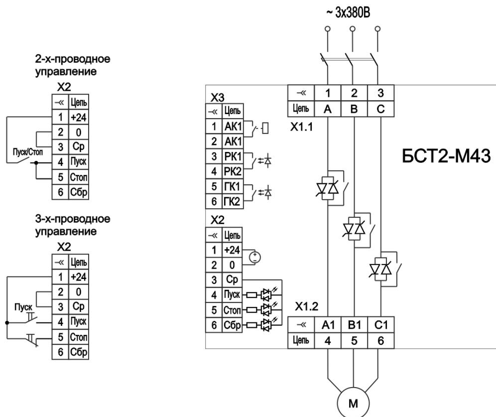
Рисунок 4 – Пример схемы подключения БСТ2-М43
