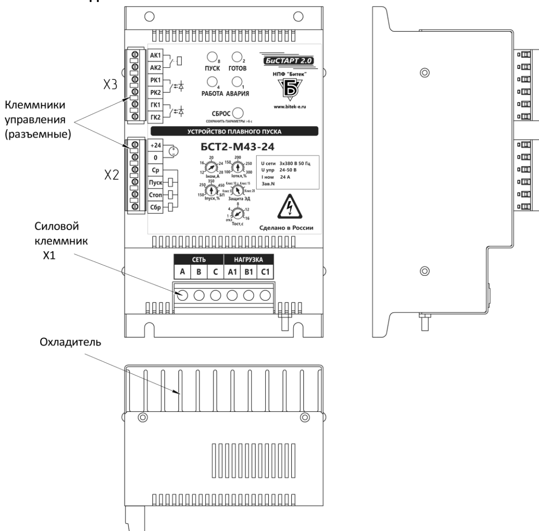
Рисунок 1 - Внешний вид пускателя БСТ2-М43-24
