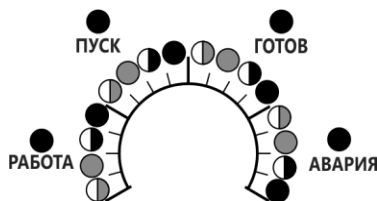
Рисунок 7 Индикация положения потенциометра
