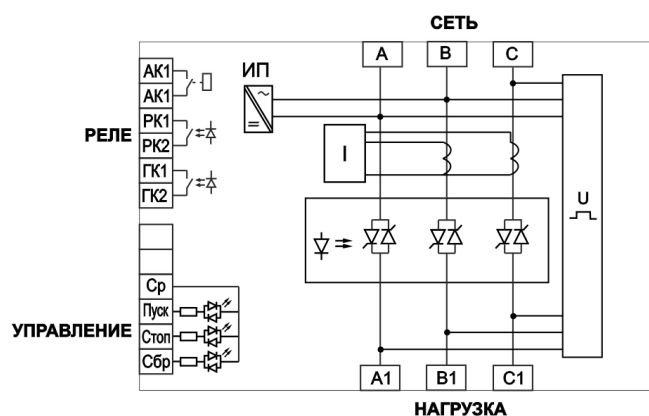
а) БСТ2-Н40, БСТ2-Н41, БСТ2-Н42
