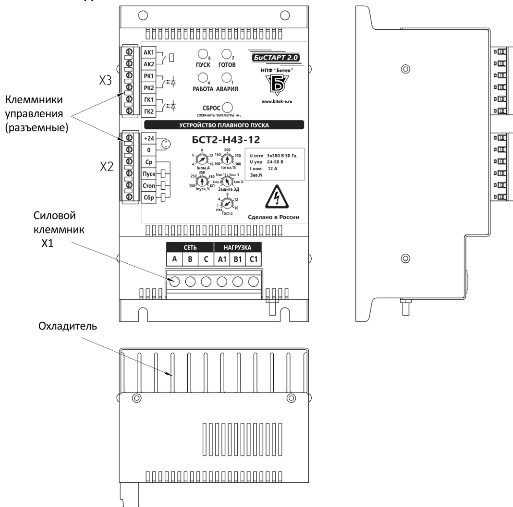
Рисунок 1 - Внешний вид пускателя БСТ2-Н43-12
