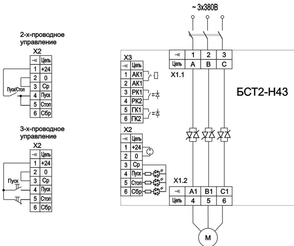
Рисунок 4 – Пример схемы подключения БСТ2-Н43
