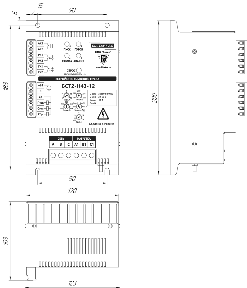
Рисунок А.1 – Габаритно-установочные размеры БСТ2-...-12
