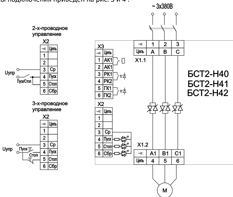
Рисунок 3 – Пример схемы подключения БСТ2-Н40, БСТ2-Н41, БСТ2-Н42
