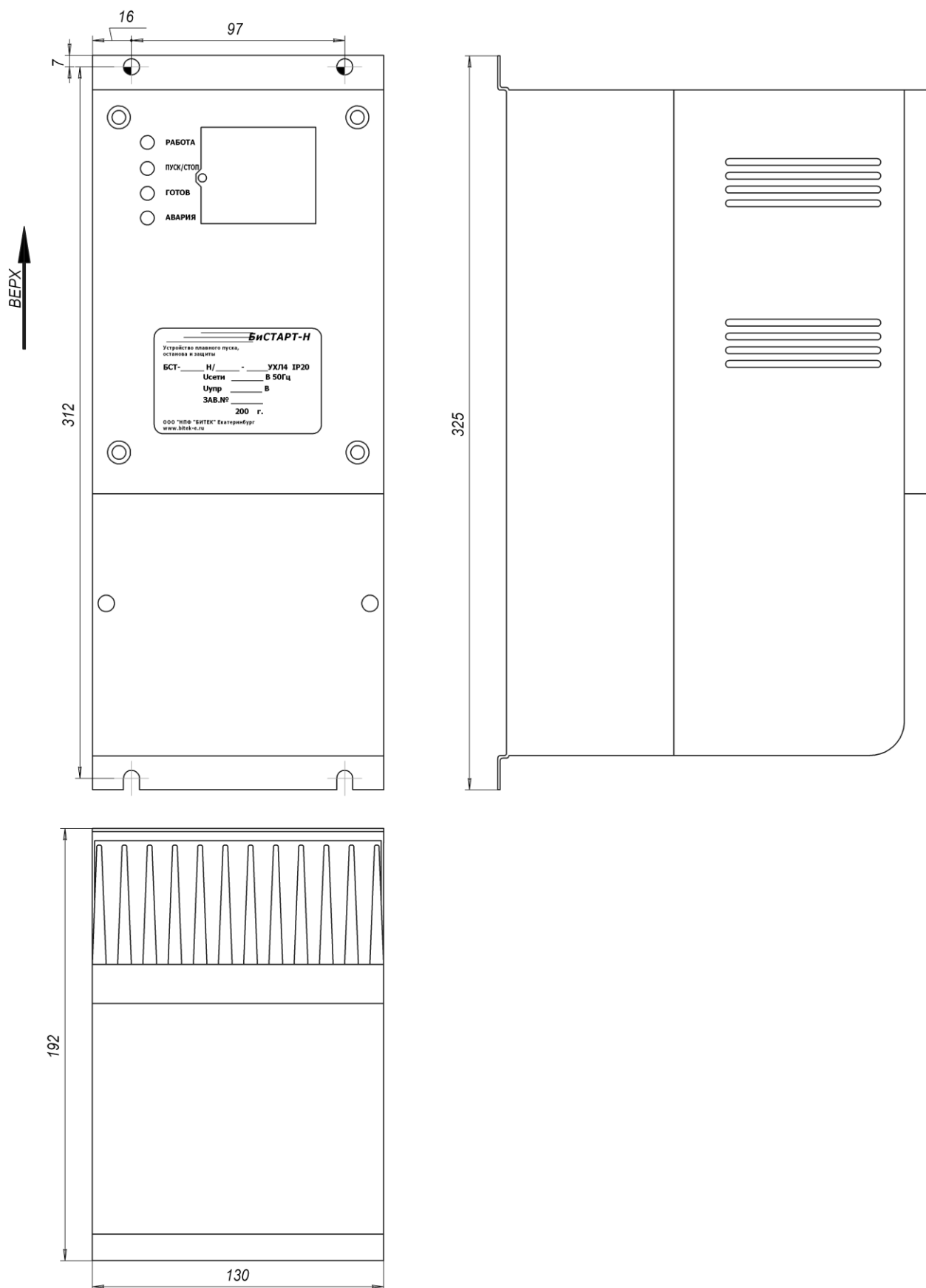
Рисунок 9 – Габаритные размеры БСТ-30Н..БСТ-60Н
