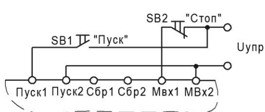
Рисунок 2 – Схема подключения пускателя
