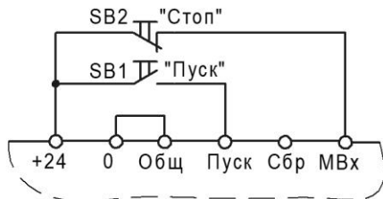
Рисунок 2 – Схема подключения пускателя
