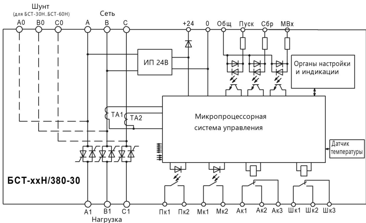
Рисунок 1 – Функциональная схема пускателя а) БСТ-ххН/380-00, БСТ-ххН/380-10, БСТ-ххН/380-20 б) БСТ-ххН/380-30
