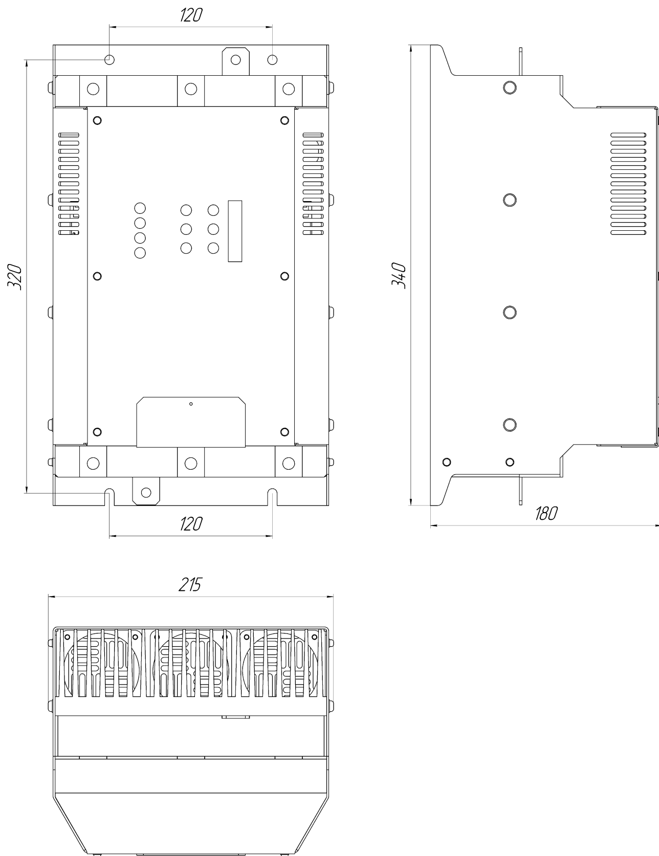
Рисунок 10 – Габаритные размеры БСТ-75Н..БСТ-110Н
