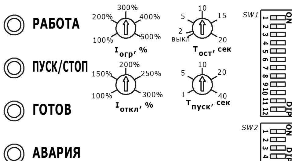
Рисунок 4 – Органы настройки пускателя
