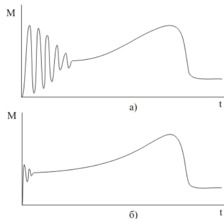
Рисунок 5 – Электромагнитный момент двигателя при прямом (а), и пофазном (б) пуске
