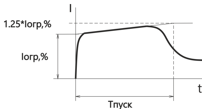
Рисунок 6 – Плавный пуск с ограничением тока
