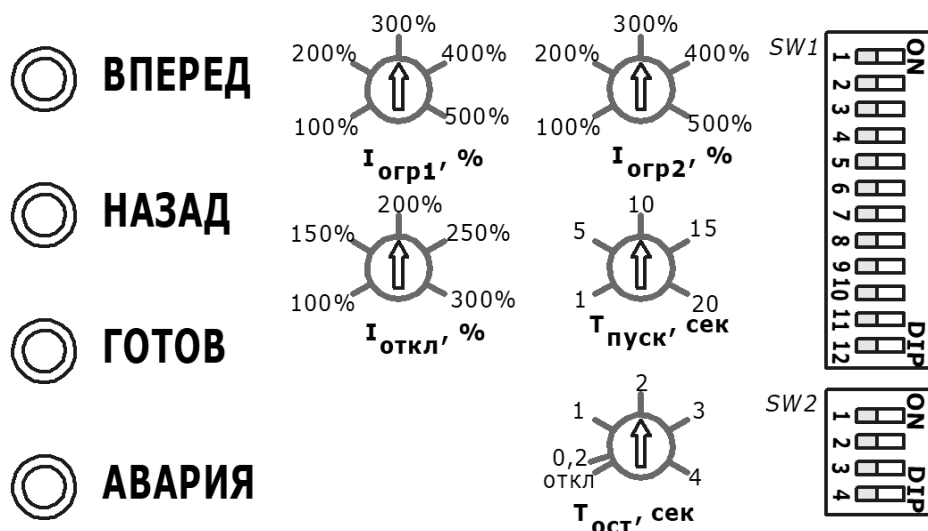
Рисунок 3 – Органы настройки пускателя
