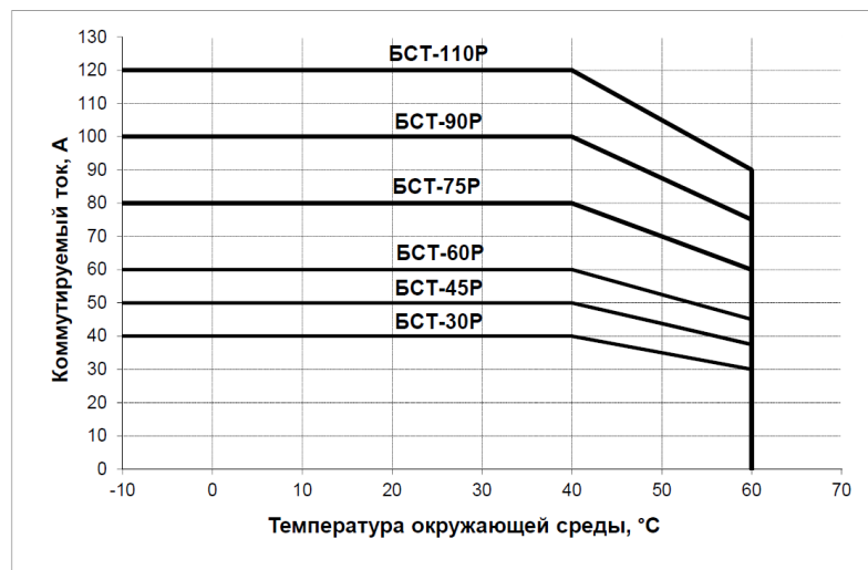
Рисунок 12 – Зависимость коммутируемого тока от температуры окружающей среды:
