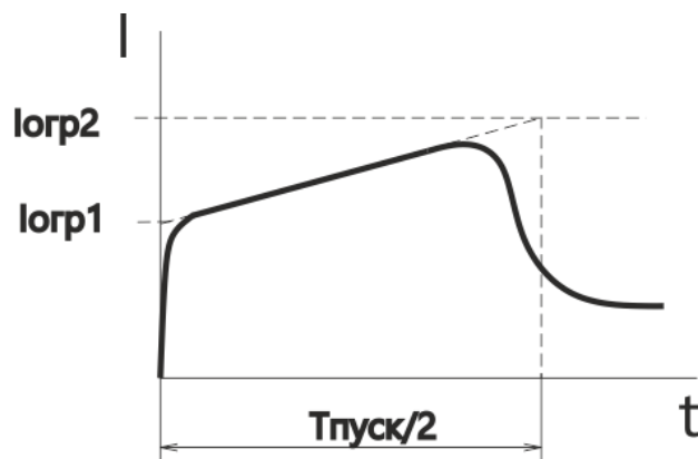
Рисунок 5 – Плавный пуск с нарастанием тока
