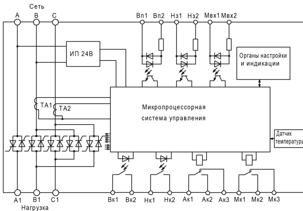
а) БСТ-ххР/380-00Т, БСТ-ххР/380-10Т и БСТ-ххР/380-20Т
