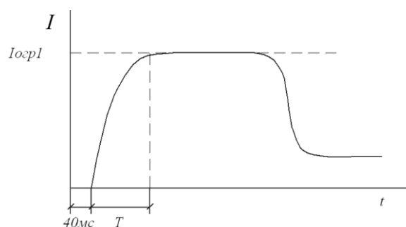
Рисунок 5 – Плавный пуск с ограничением тока
