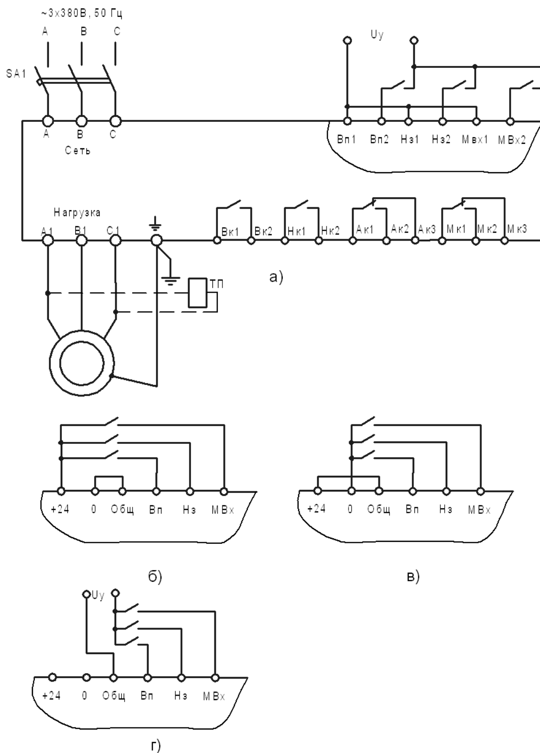
Рисунок 2 – Схема подключения пускателя
