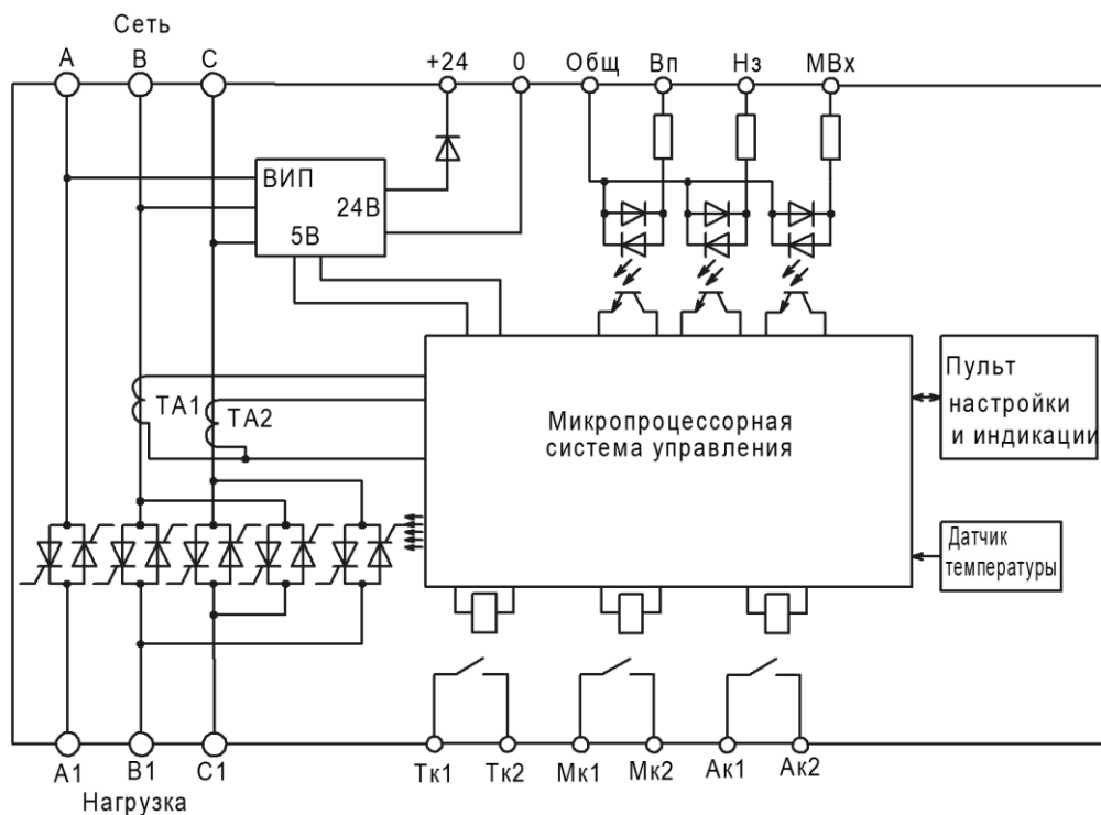
б) БСТ-xxP/xx-30K
