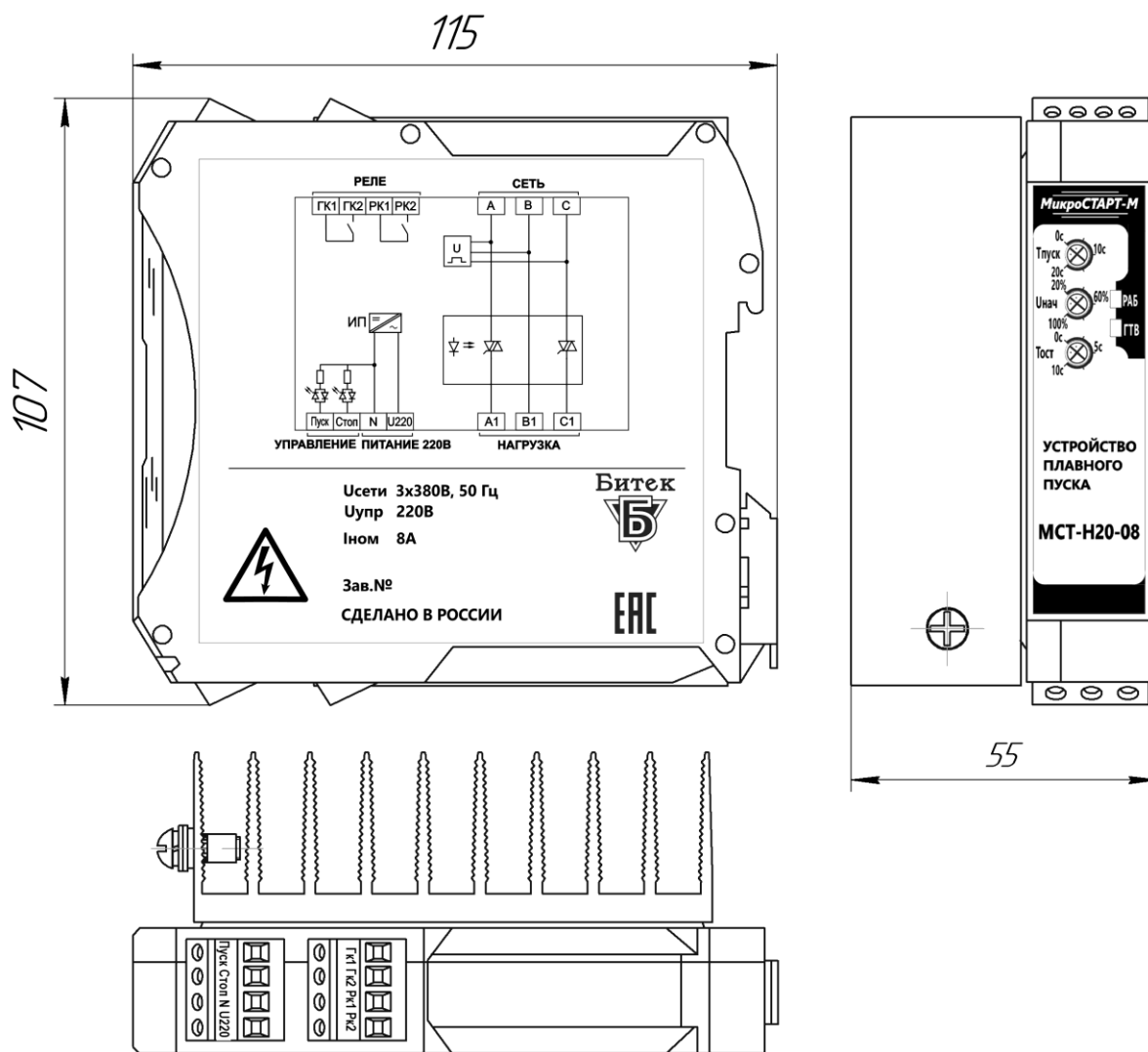
Рисунок А.2 – Габаритно-установочные размеры МСТ-H2x-08
