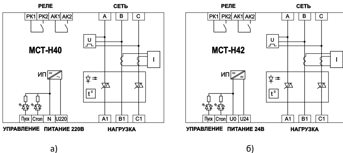
Рисунок 2 – Функциональная схема пускателей а) МСТ-Н40-хх, б) МСТ-Н42-хх
