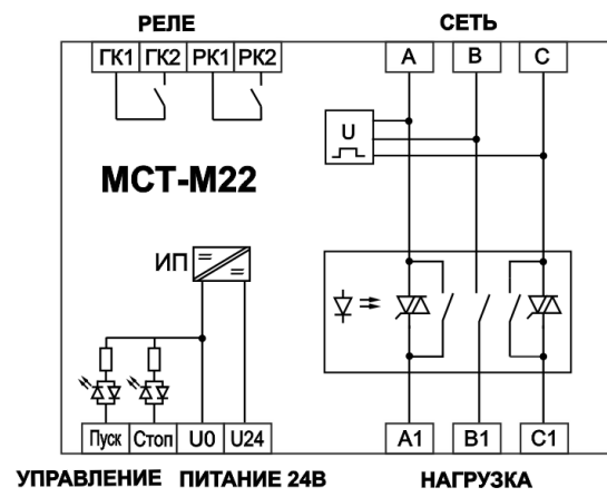
Рисунок 2 – Функциональная схема пускателей а) МСТ-M20-xx, б) МСТ-M22-xx
