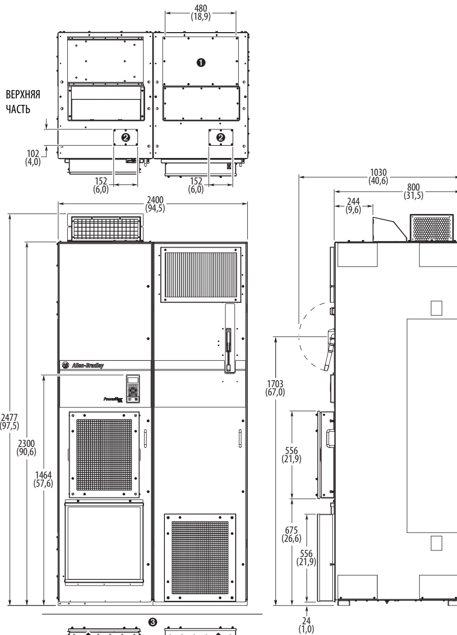
Рис. 49 - IP54, NEMA 12, шкаф исполнения ЦУЭД, типоразмер 8 (коды корпуса K и Y) IP54, UL тип 12, шкаф исполнения ЦУЭД, типоразмер 8 (код корпуса J) (привод глубиной 800 мм с отсеком дополнительного оборудования шкафа)
