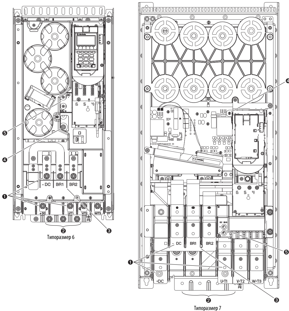
Рис. 81 - Расположение точек подключения и силовых клемм у типоразмеров 6 и 7 с общим входом постоянного тока
