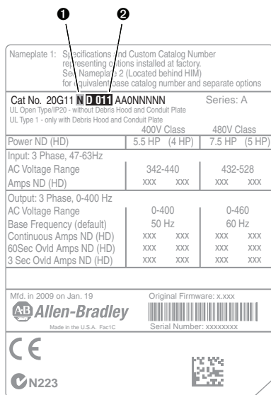
Паспортная табличка привода 1, типоразмеры 1–7
