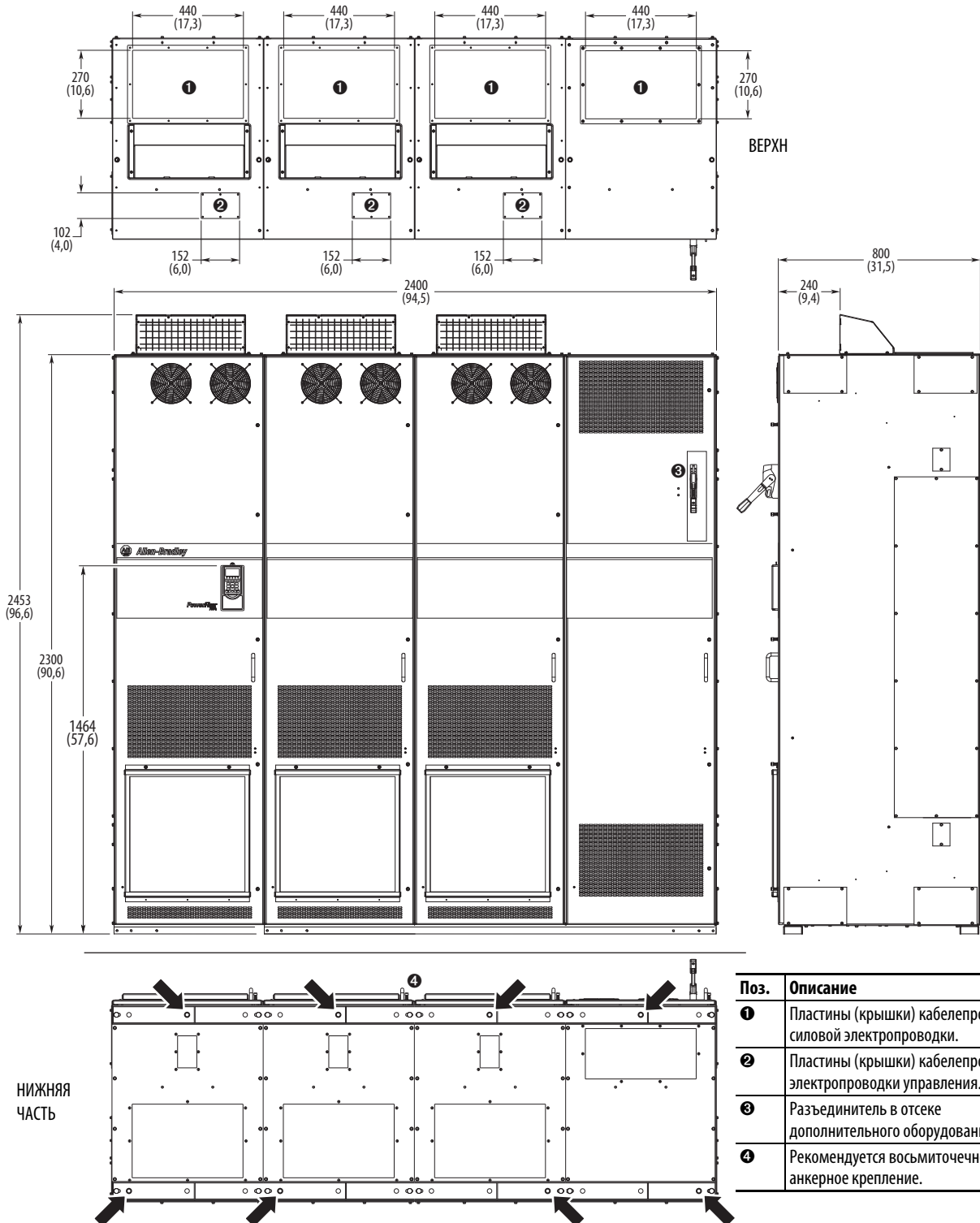
Рис. 65 - IP20, NEMA/UL тип 1, шкаф исполнения ЦУЭД, типоразмер 10 (коды корпуса L, P, W - привод глубиной 800 мм и отсек дополнительного оборудования шкафа)
