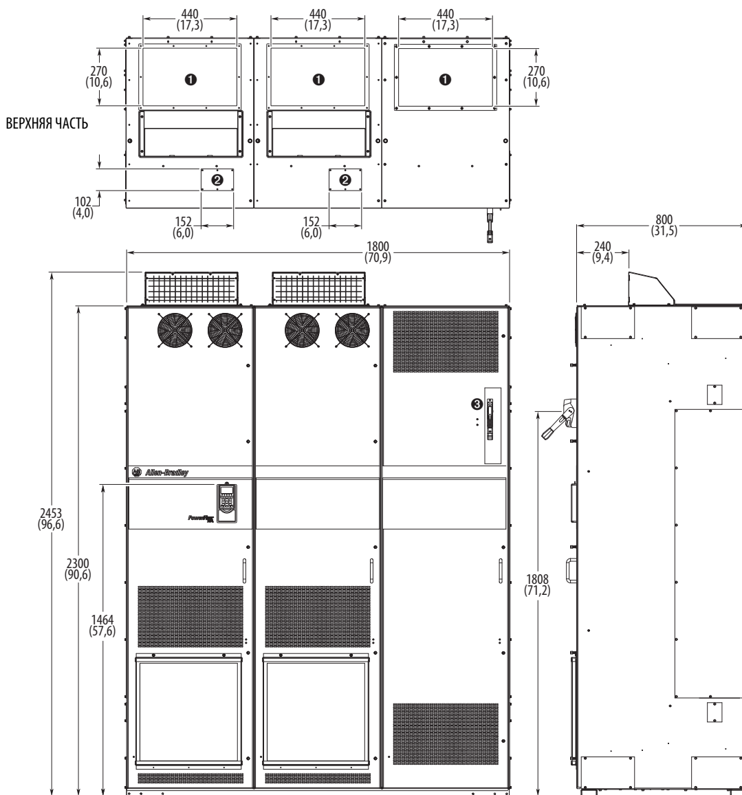
Рис. 55 - IP20, NEMA/UL тип 1, шкаф исполнения ЦУЭД, типоразмер 9 (коды корпуса L, P, W - привод с отсеком дополнительного оборудования шкафа глубиной 800 мм)
