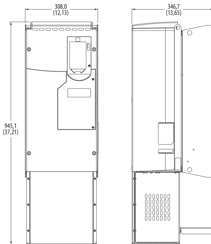
Рис. 28 - Комплект NEMA/UL тип 1, типоразмер 6
