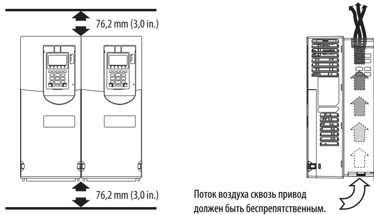
Рис. 11 - Минимальные монтажные зазоры для типоразмеров 1–7
