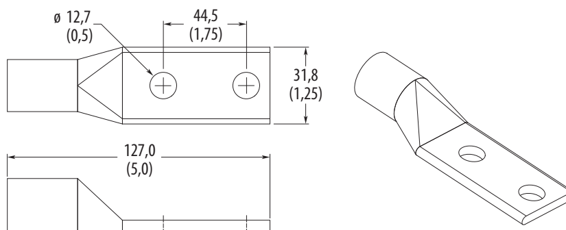
Рис. 87 - Стандартные обжимные наконечники: приблизительные максимальные размеры
