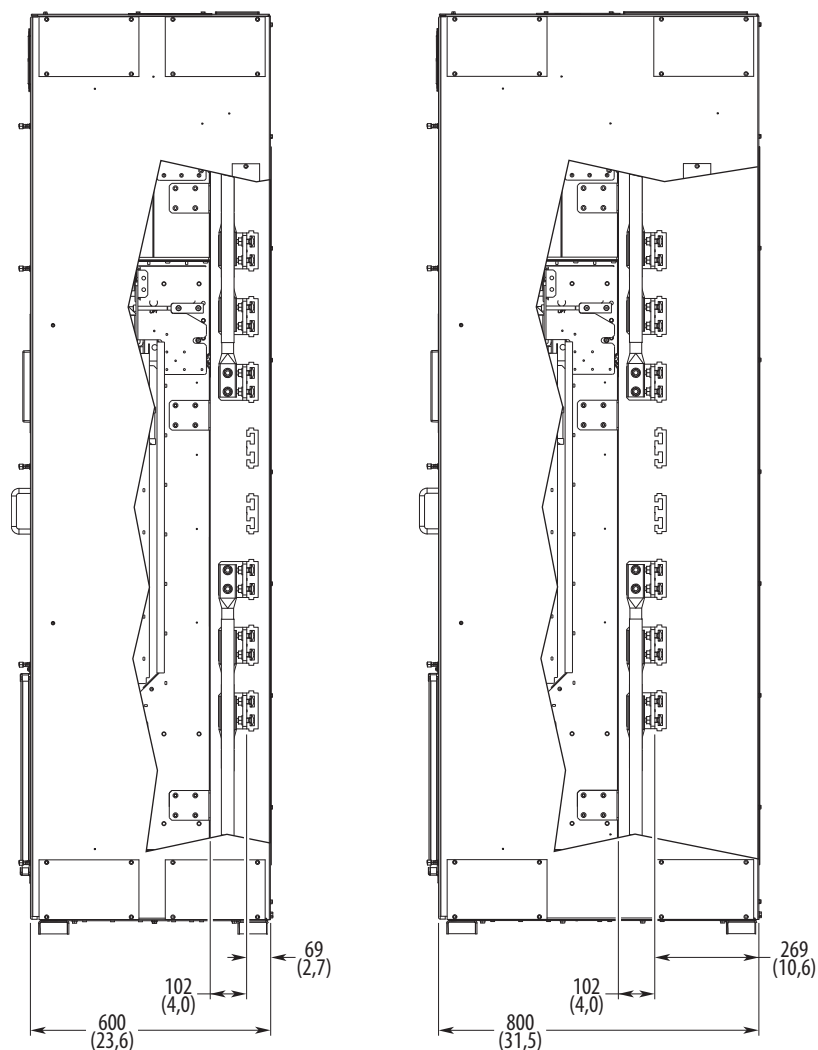
Рис. 91 - Зазоры шкафа
