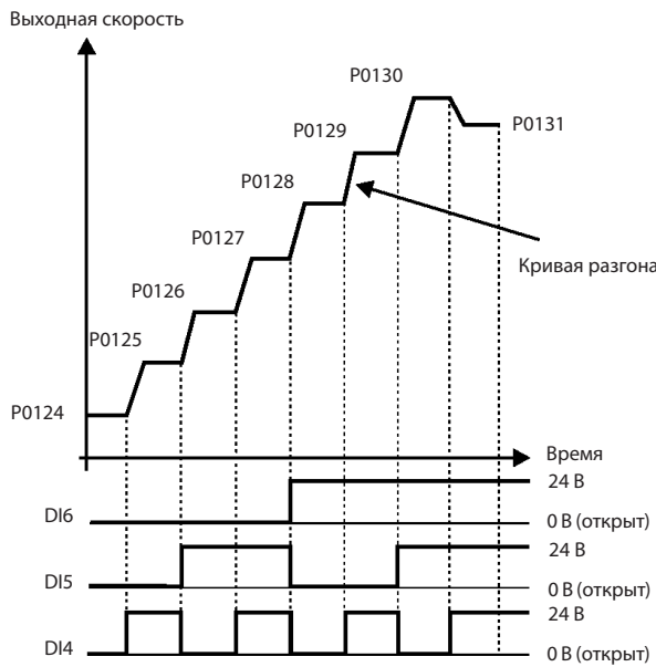
Рис. 12.4. Многоскоростной режим
