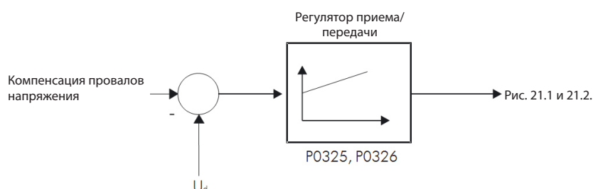
Рис. 21.3. ПИ-регулятор компенсации провалов
