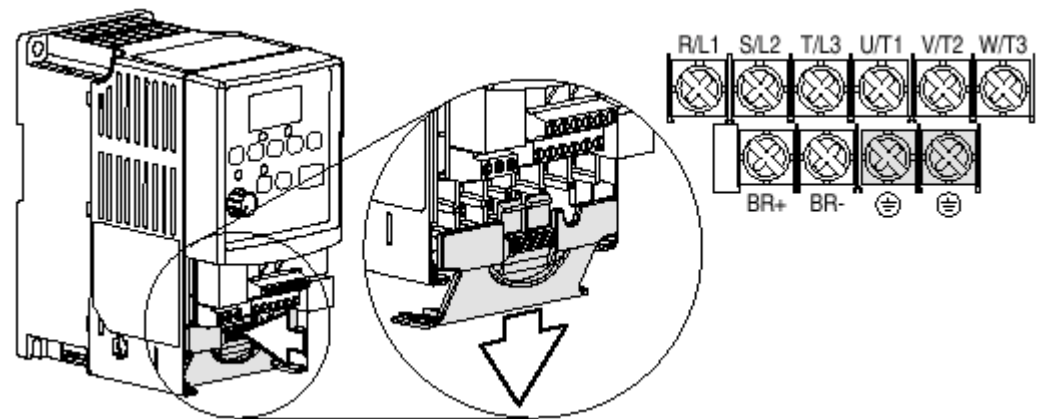
Рис.1.4 Силовой клеммный блок (Показан типоразмер А)
