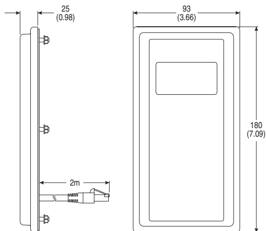
Рис. Б.13 Удаленный сокращенный модуль НИМ (крепление на панели). Размеры указаны в миллиметрах (в скобках даны значения в дюймах). Номер по каталогу: 22-НМ-C2S
